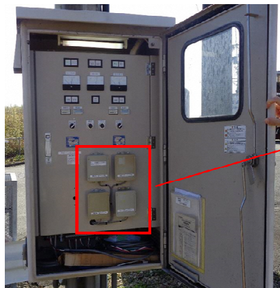
※ マンホールポンプ施設の無線端末機 (NCU) と電力スマートメーターが送受信
