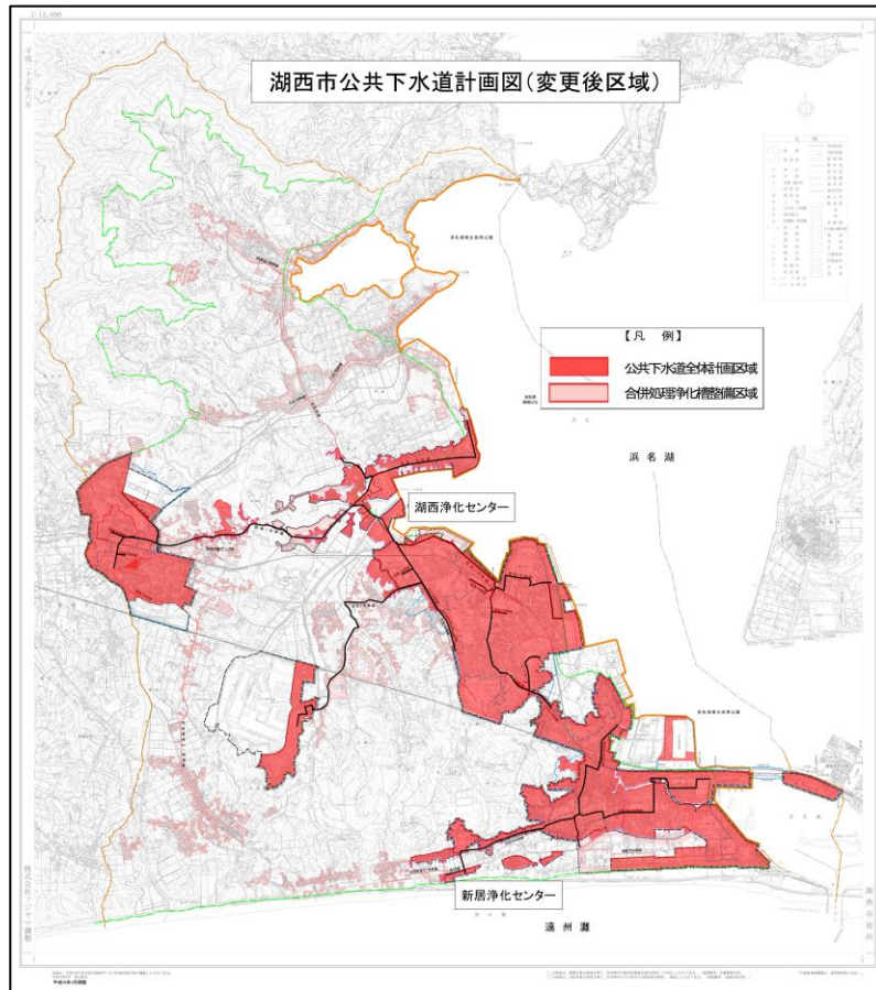
図 2-3 下水道計画一般図
