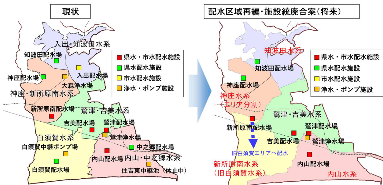
図 3-2 配水区域再編・施設統廃合イメージ
