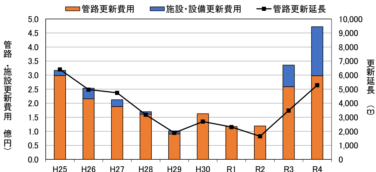
図 2-2 管路・施設の更新費用及び管路更新延長の推移
