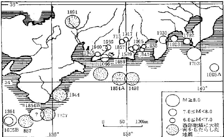
県西部地域に被害を与えた主な地震の震央
