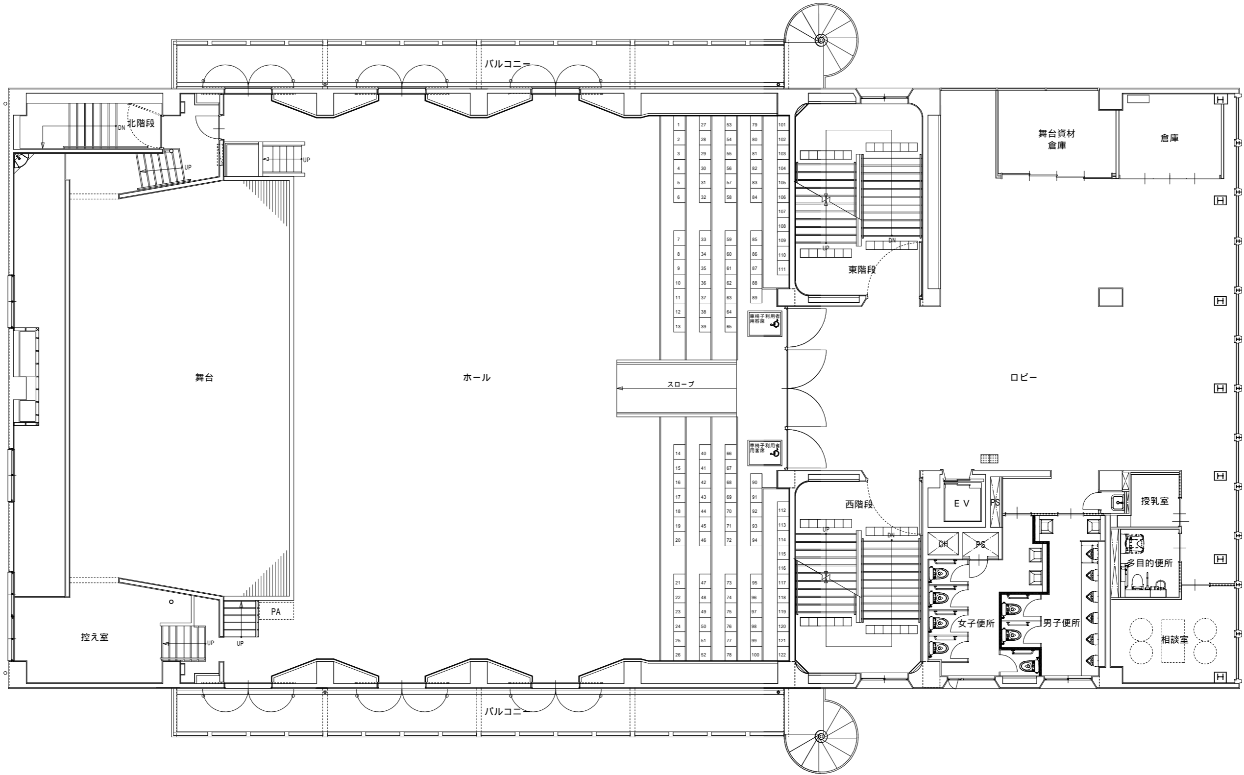
3階平面図
