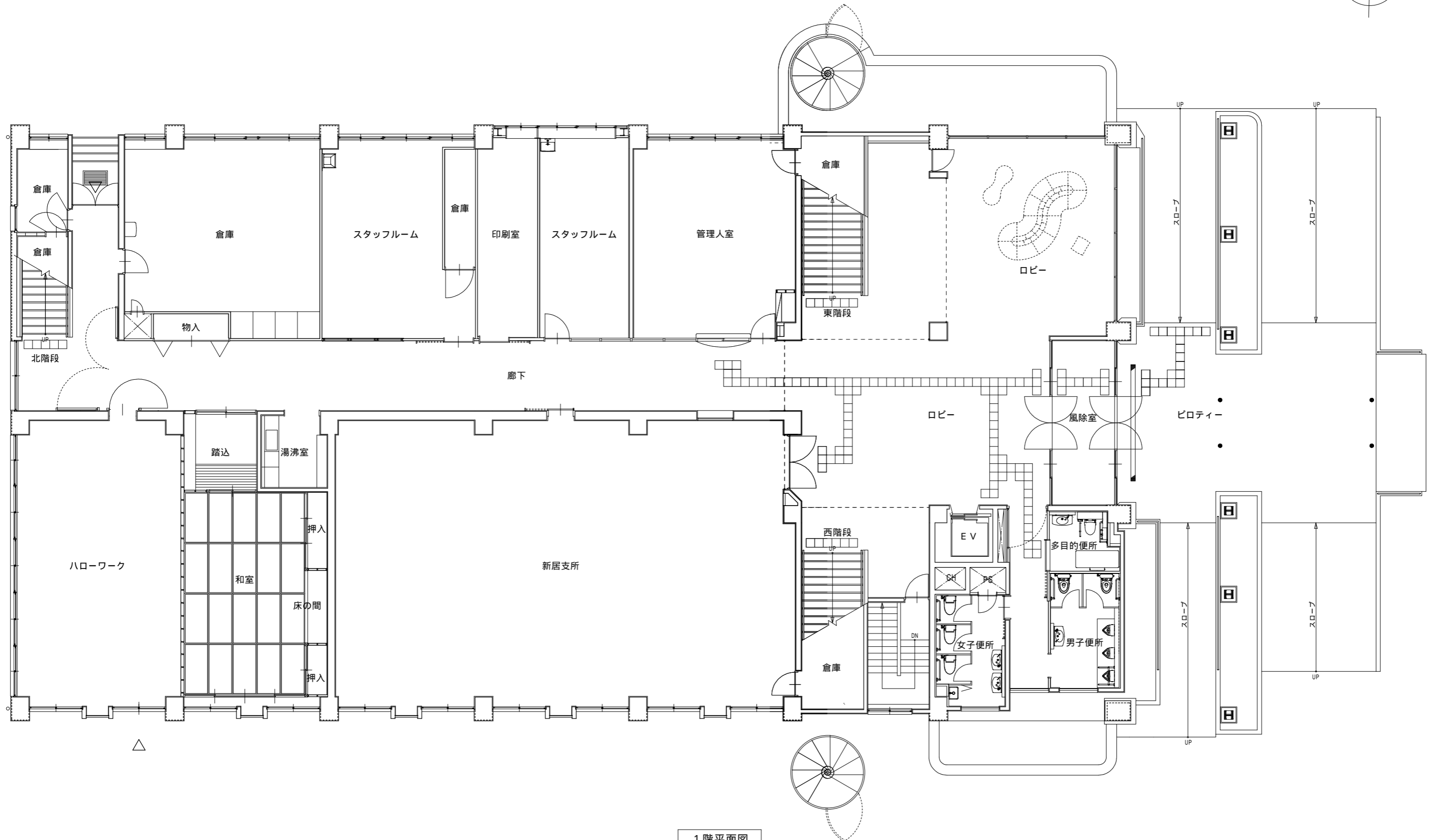
1階平面図
