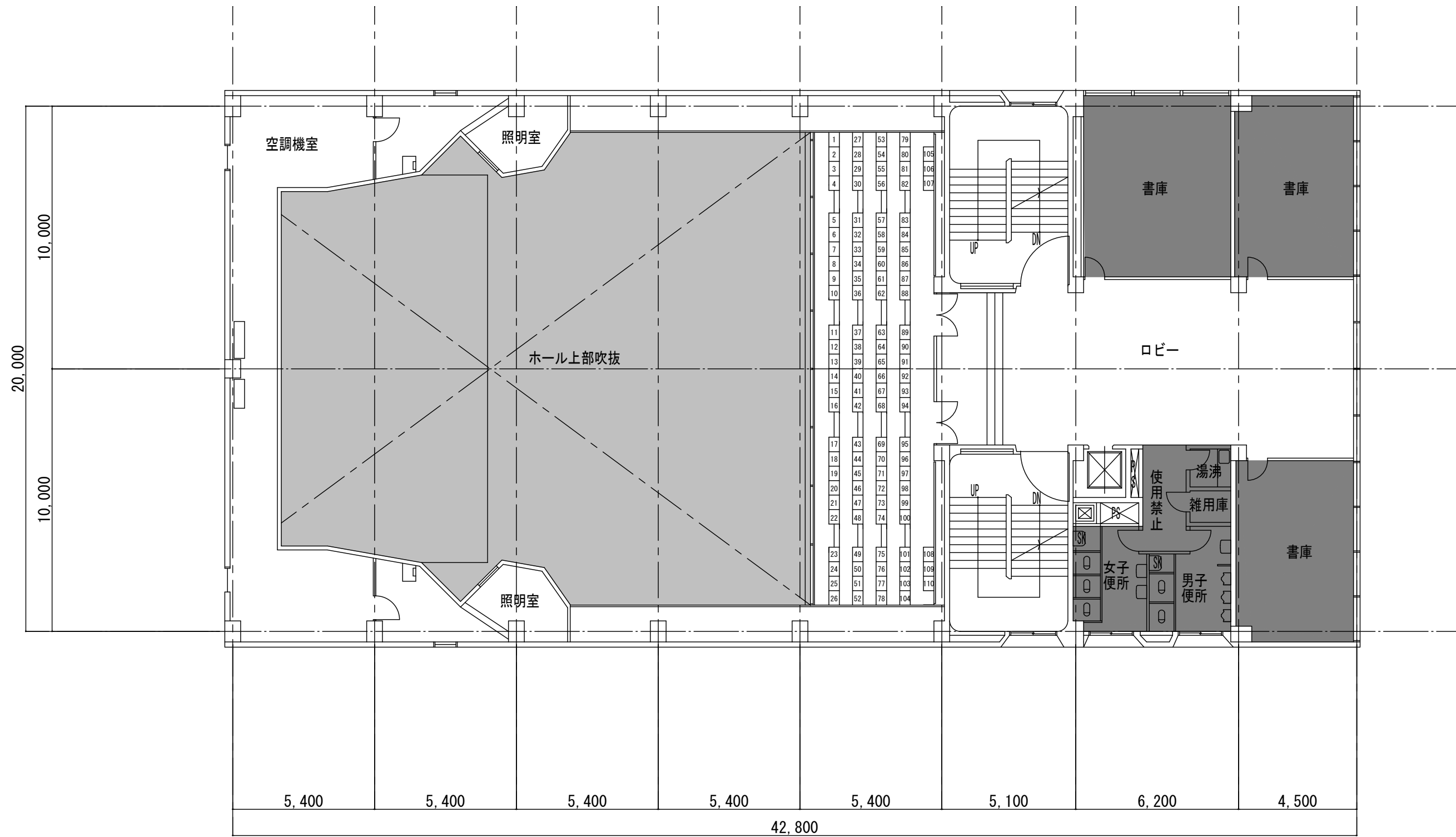
4階平面図
