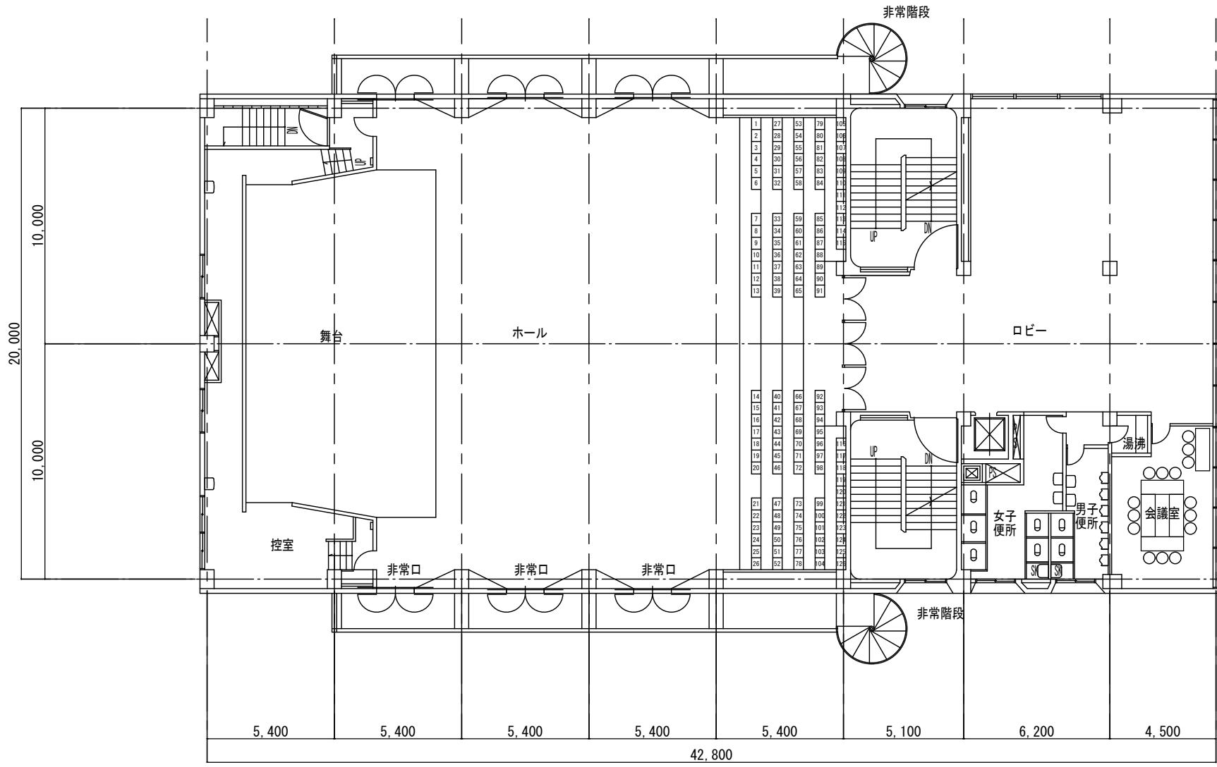
3階平面図
