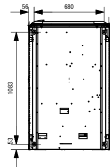
底面図
