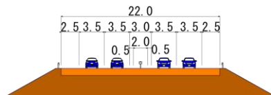
高上式(土工部)
