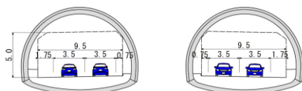
地下式(トンネル部)
