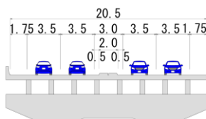
高上式(橋梁部)
